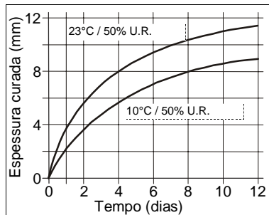
Diagrama: Velocidade cura Sikaflex®-227
